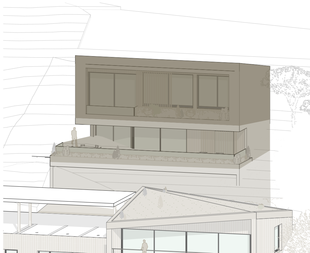
Axonométrie
